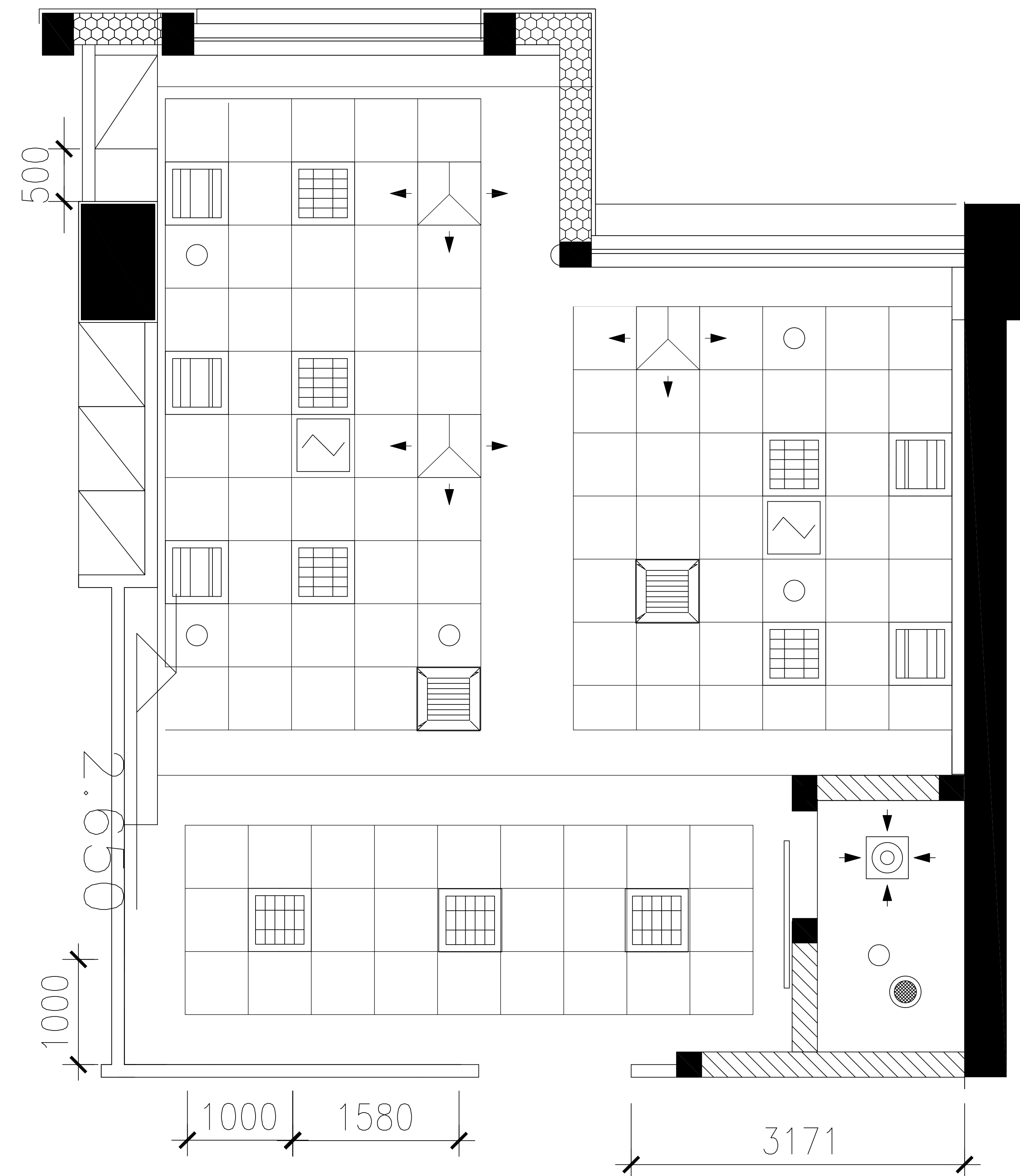
改造后图纸
