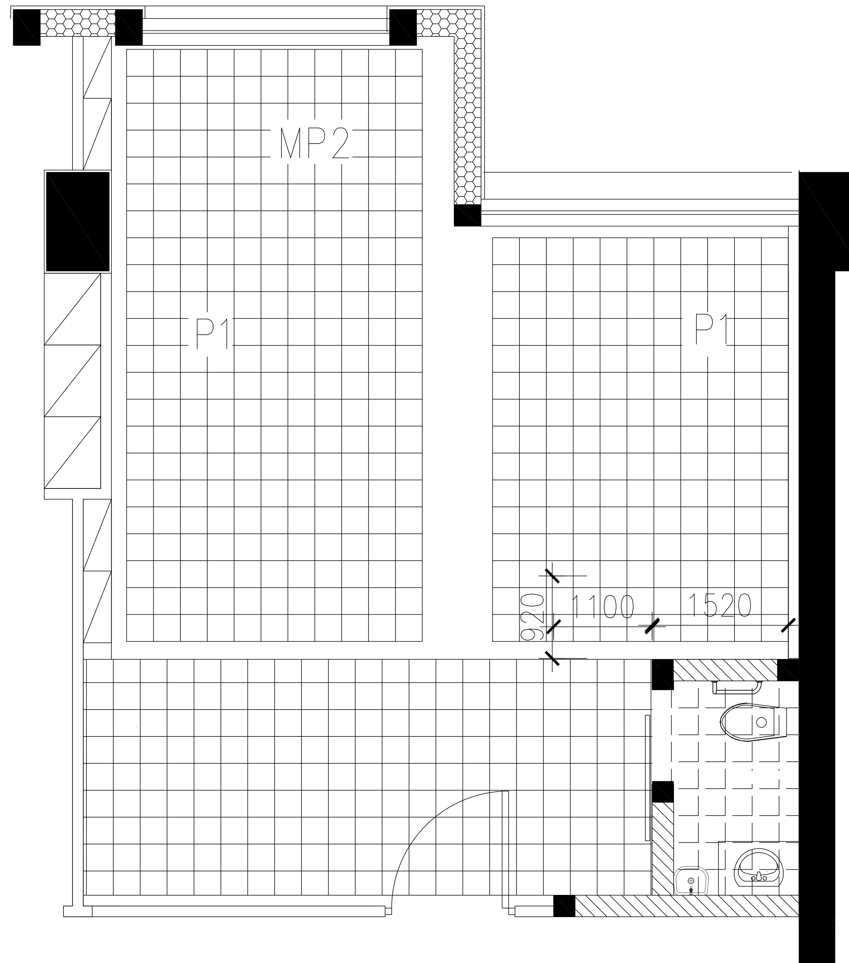
改造后地坪图
