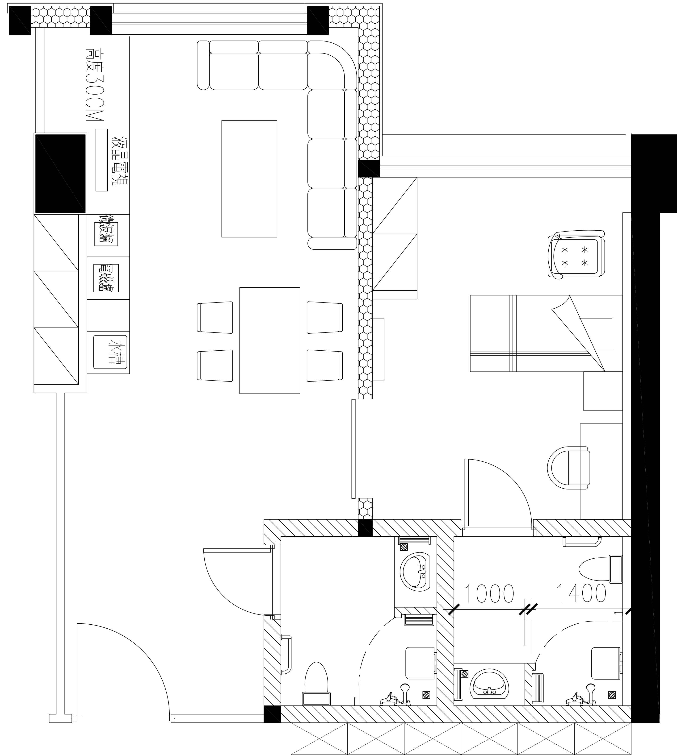
原平面图
