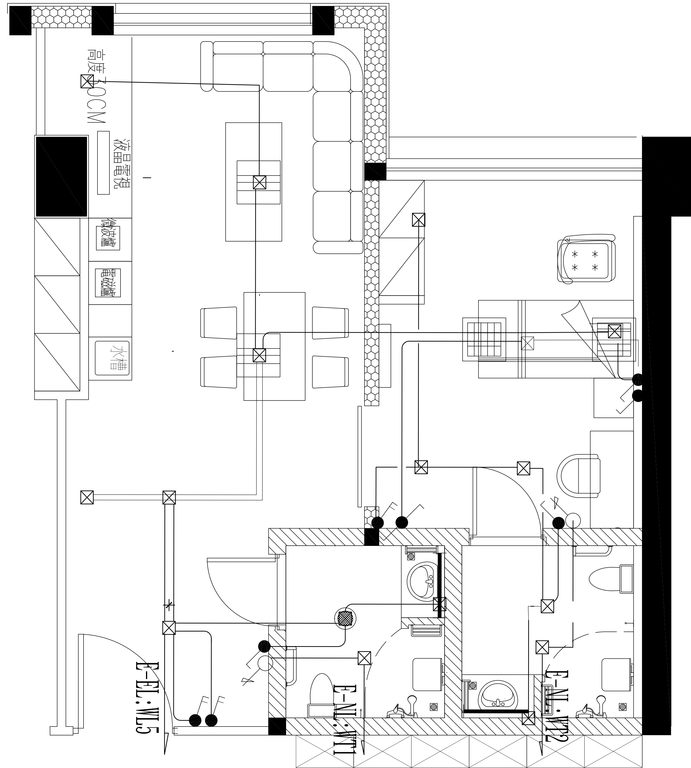
原平面图
