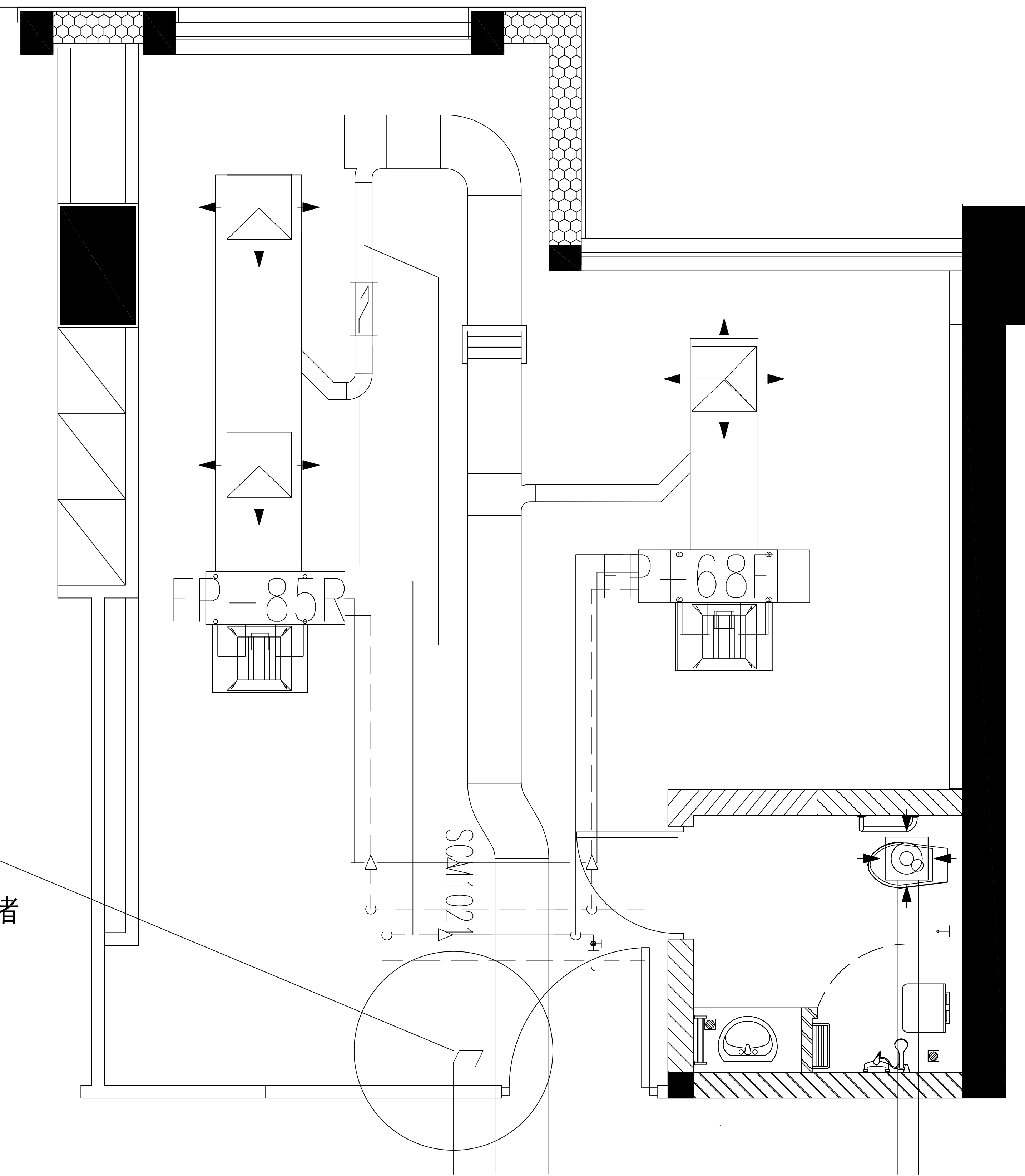
改造后通风图
