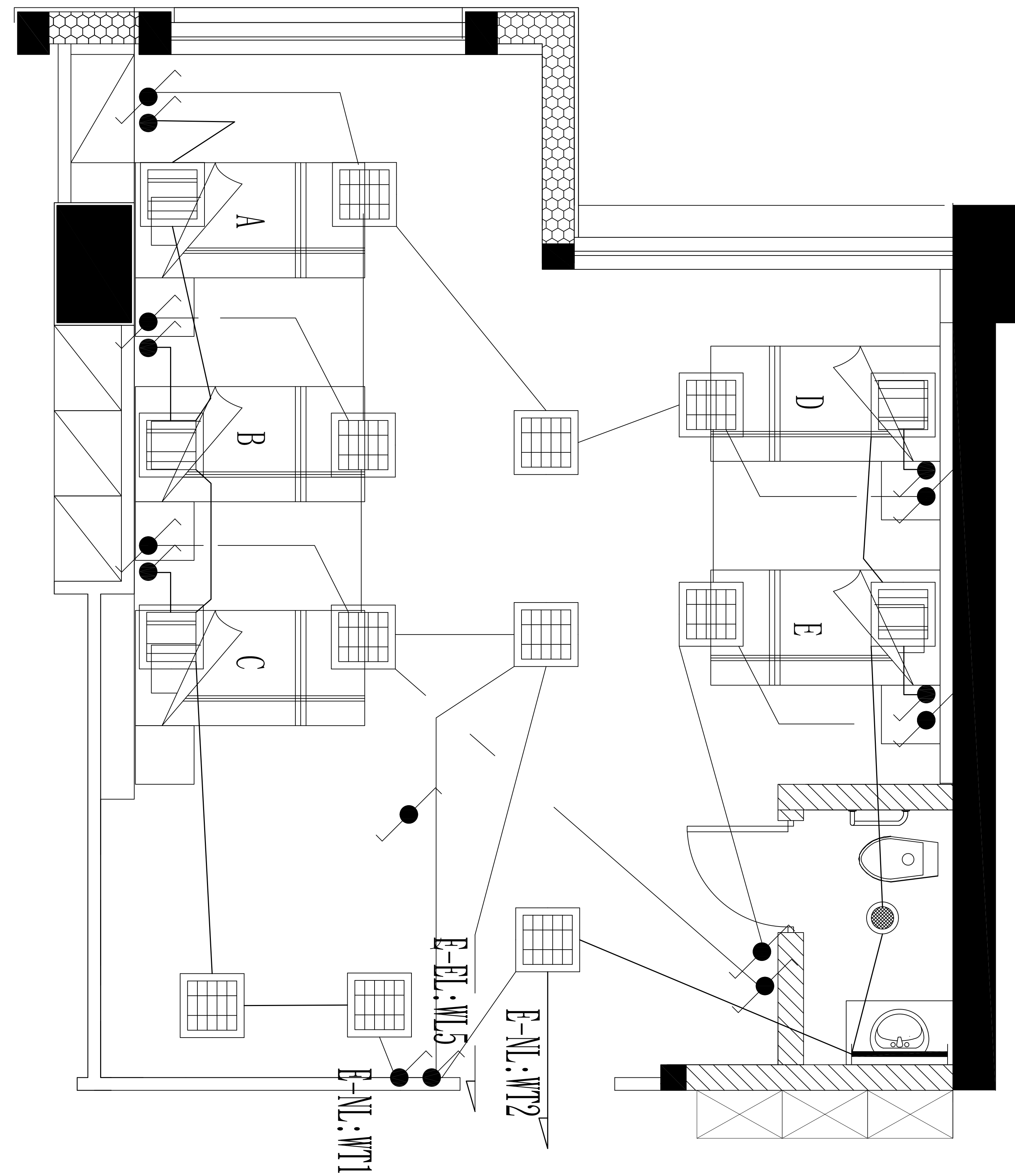
5床图纸
