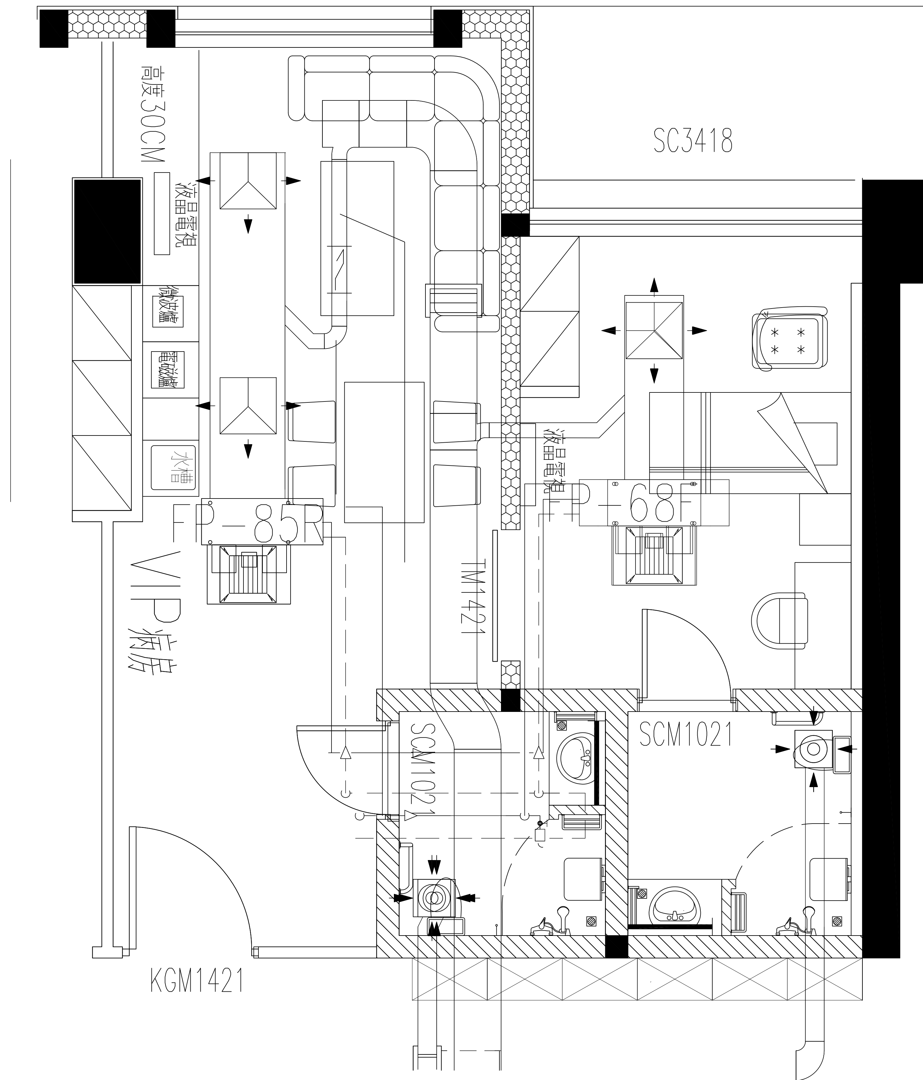
原通风图
