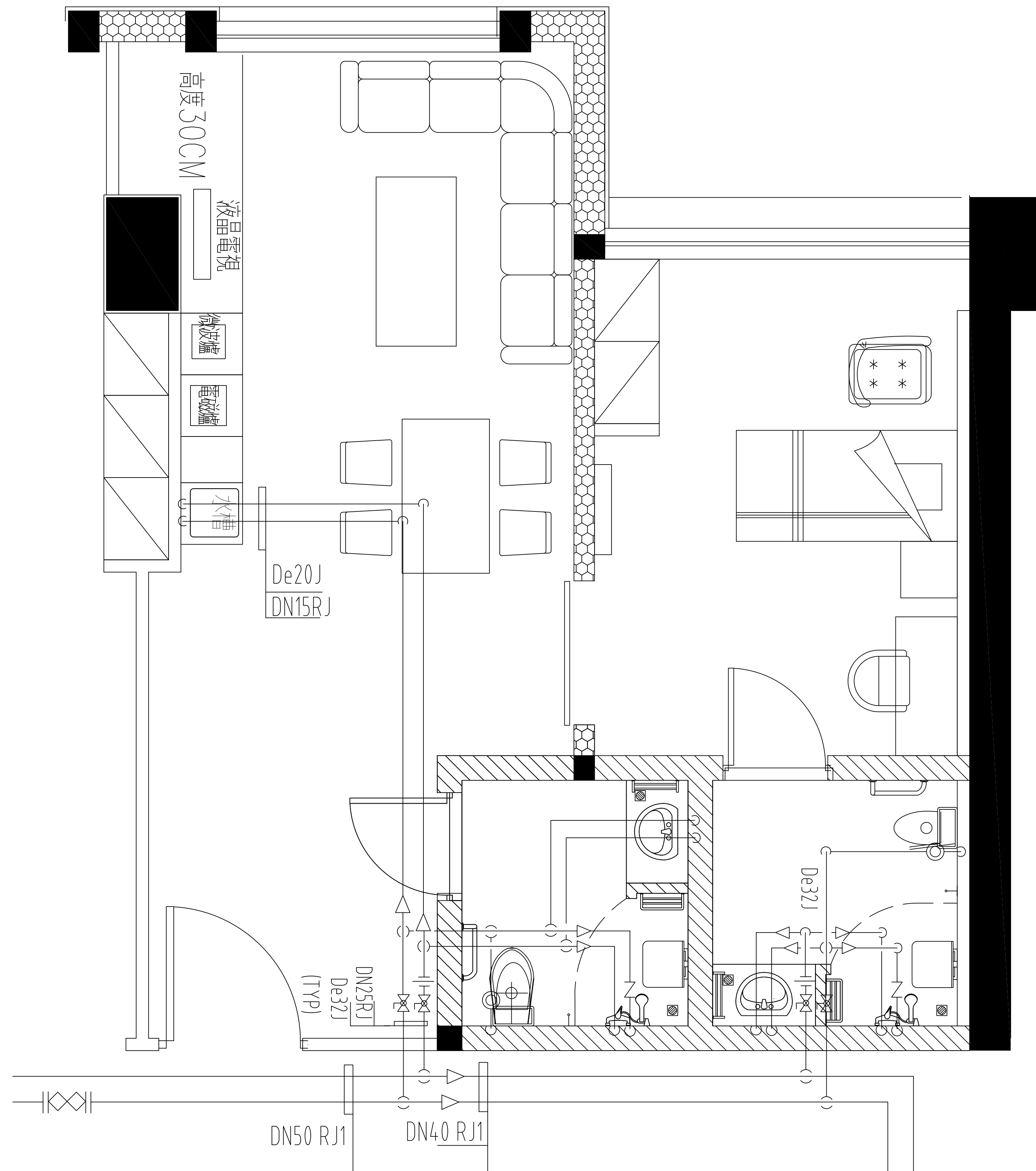
原平面图
