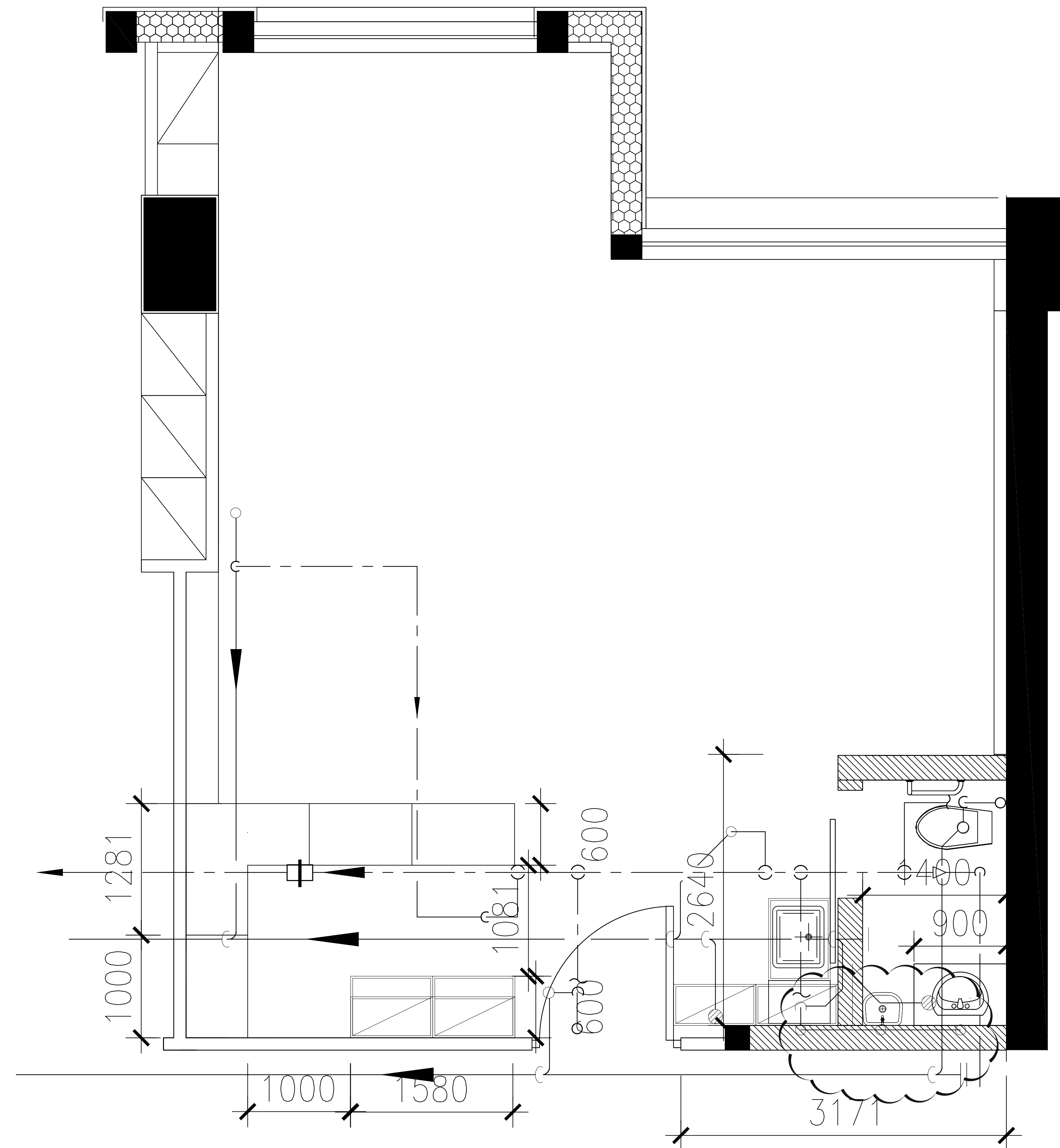
5床图纸
